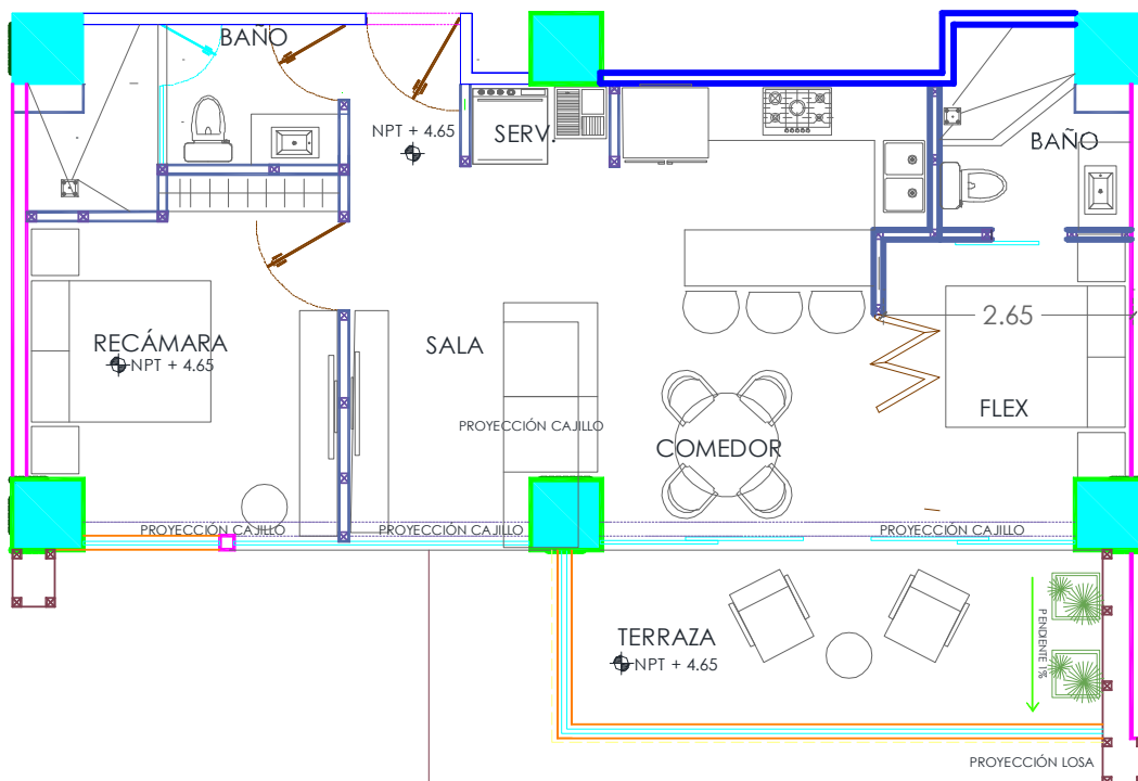
Planta Arquitectónica
