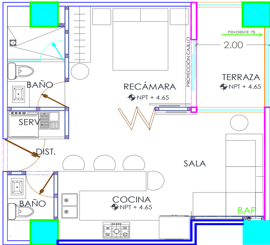
Planta Arquitectónica
