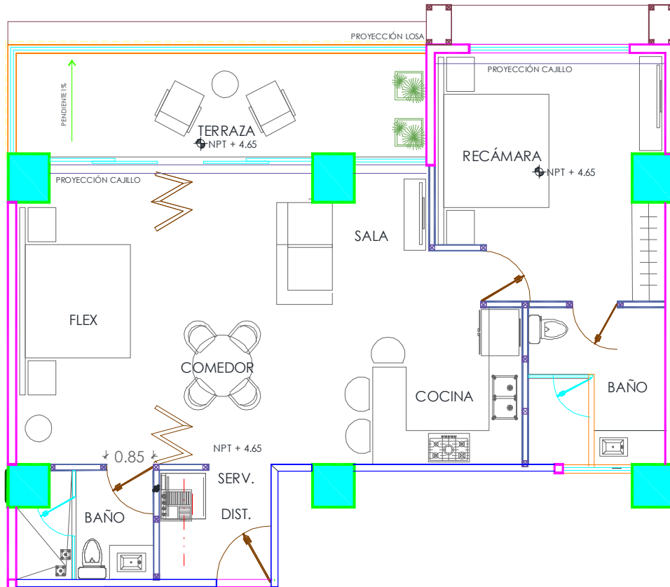
Planta Arquitectónica
